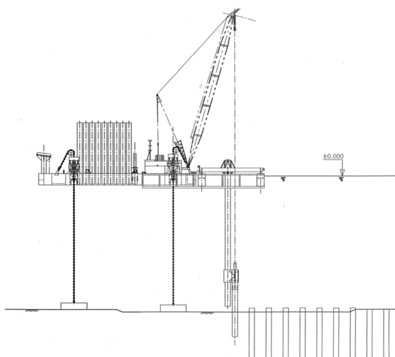
FIG. 20. Tension-leg barge
